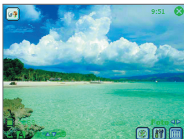
Fotomodus
