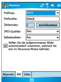
Kameraoptionen, Bild
