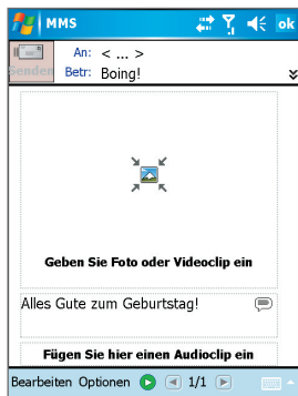
Neue MMS-Nachricht
