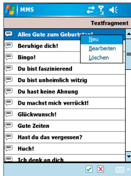
Auswahl Textfragment
