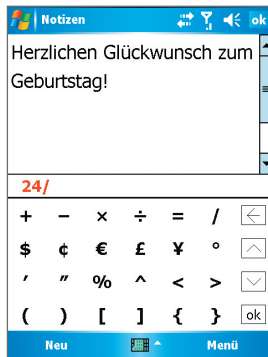
Symbolliste
