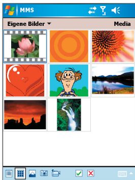
Bildschirm Medienauswahl
