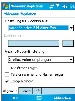
Videoanruf, Allgemein
