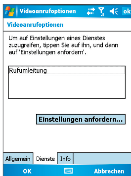
Videoanruf, Dienste
