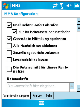
MMS konfigurieren
