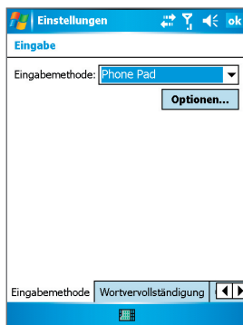
Phone Pad-Einstellungen
