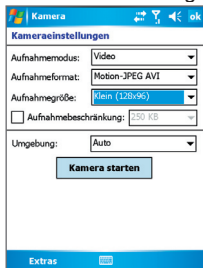
Kameraeinstellungen
